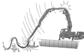
ブーム折損
